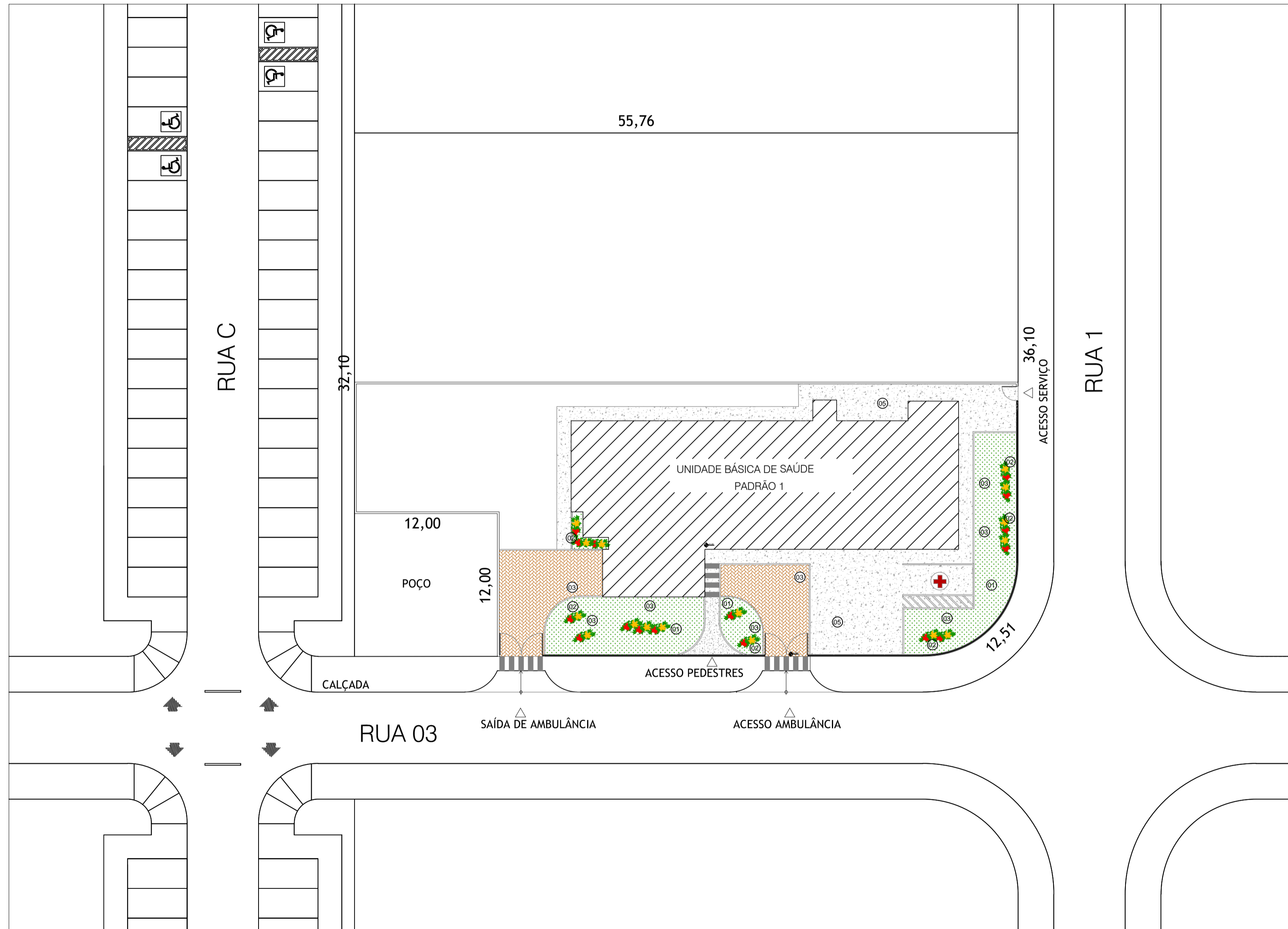
PLANTA DE PISO E PAISAGISMO ESCALA: 1/250
