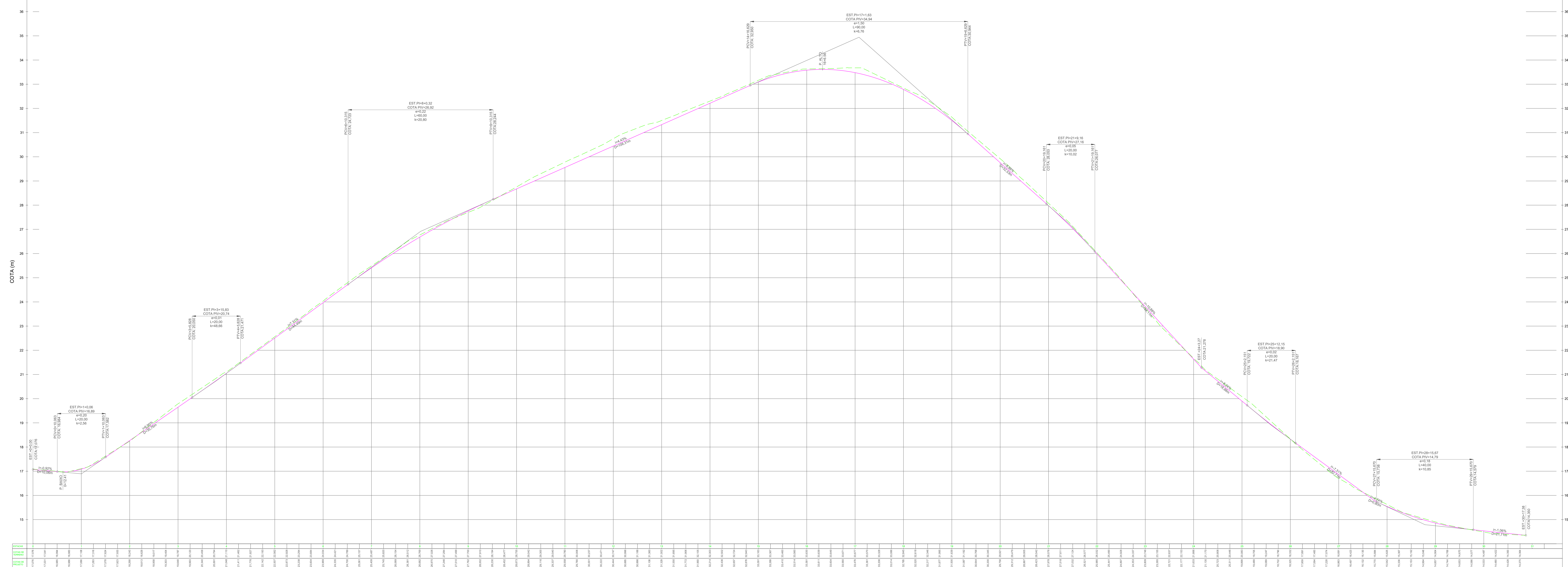
PERFIL LONGITUDINAL - Rua Treze ESC.: H:1/500 - V:1/50
