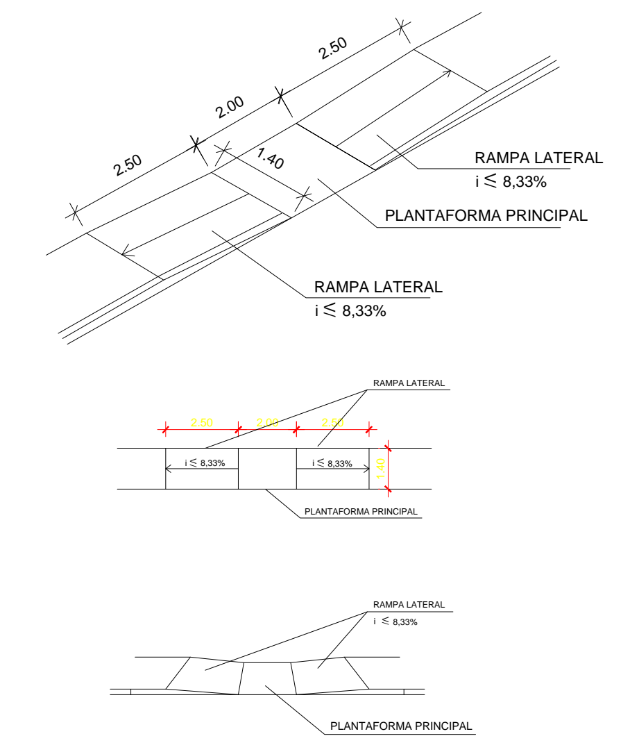
○ RAMPA PARA ACESSIBILIDADE - CALÇADA Sem escala
