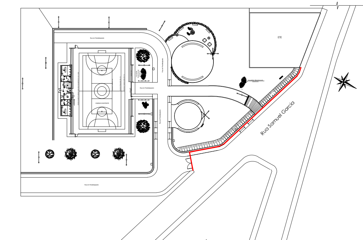
○ TAPUME Sem escala
